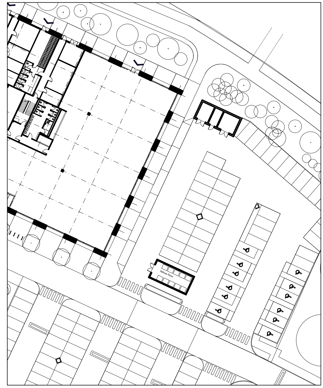
06 SITE PLAN 1:500
