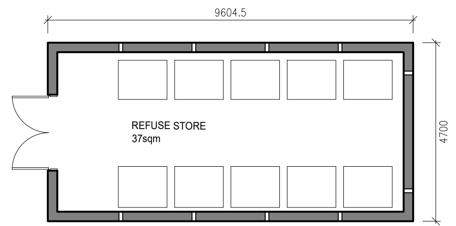
01 PLAN 1:100
